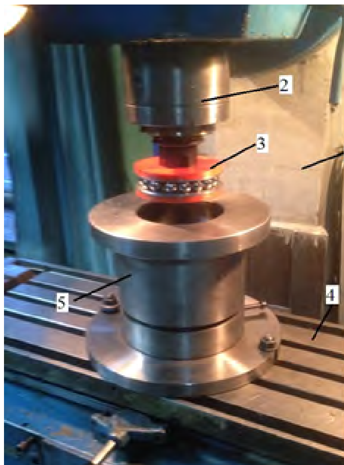
1 - вертикально-фрезерный станок; 2 - шпиндель; 3 - комбинированный инструмент; 4 - стол станка; 5 - технологическое приспособление
