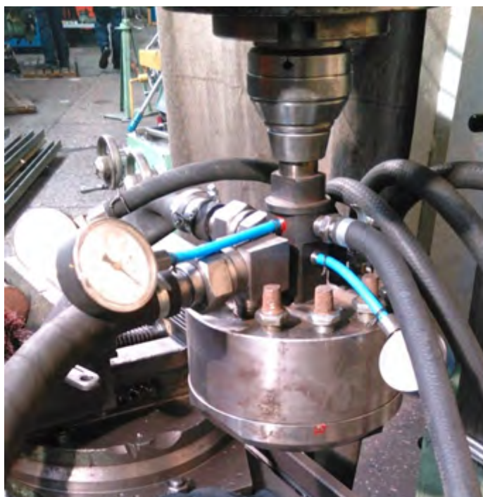
Рисунок 1 - Общий вид инструмента для упрочняющей пневмовибродинамической обработки плоских поверхностей
