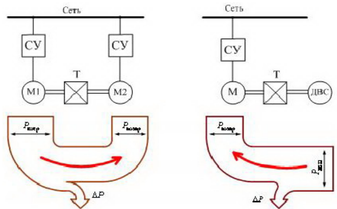
Рисунок 2 - Структурные схемы испытательных стенов
