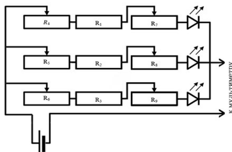
Рисунок 1 – Электрическая схема источника – RGB
